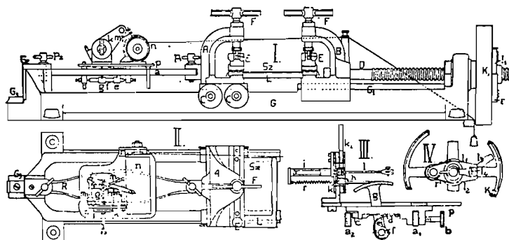
Fig. 15. Rejtő's cloth testing machine.
