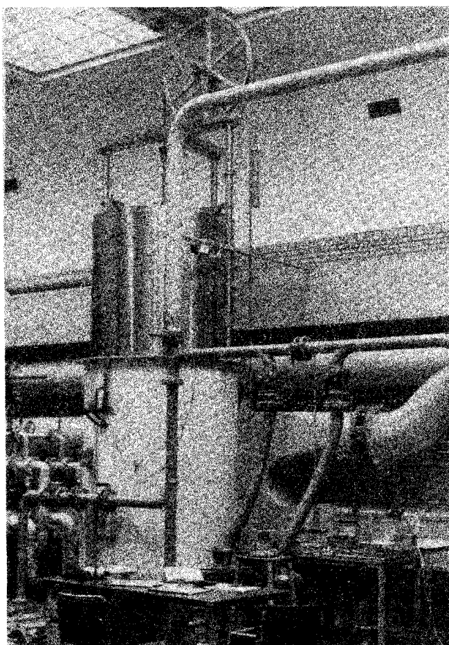
Fig. 2 Bell prover
