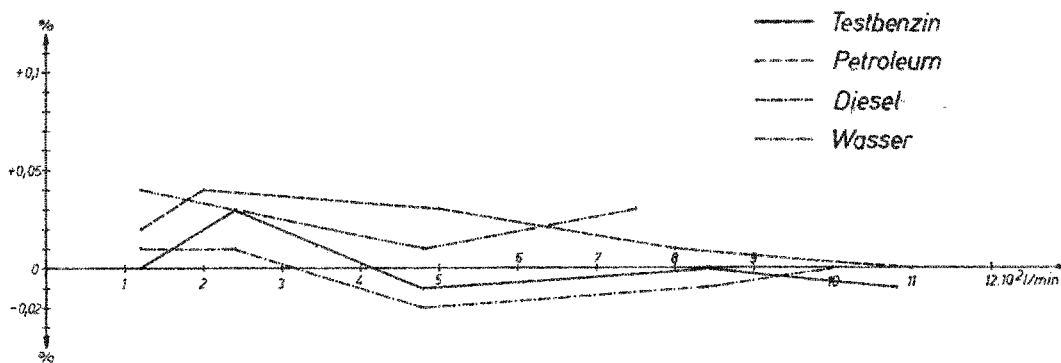
Abbildung 3: \bar{A} ..... ZÄHLERANZEIGE N_1 ..... SCHLEIFENANZEIGE N_2 ..... EICHKOLBENANZEIGE \left( \frac{\bar{A} - N_1}{N_1} \cdot 100 \right)_{\text{SCHLEIFE}} - \left( \frac{\bar{A} - N_2}{N_2} \cdot 100 \right)_{\text{EICHKOLBEN}}
